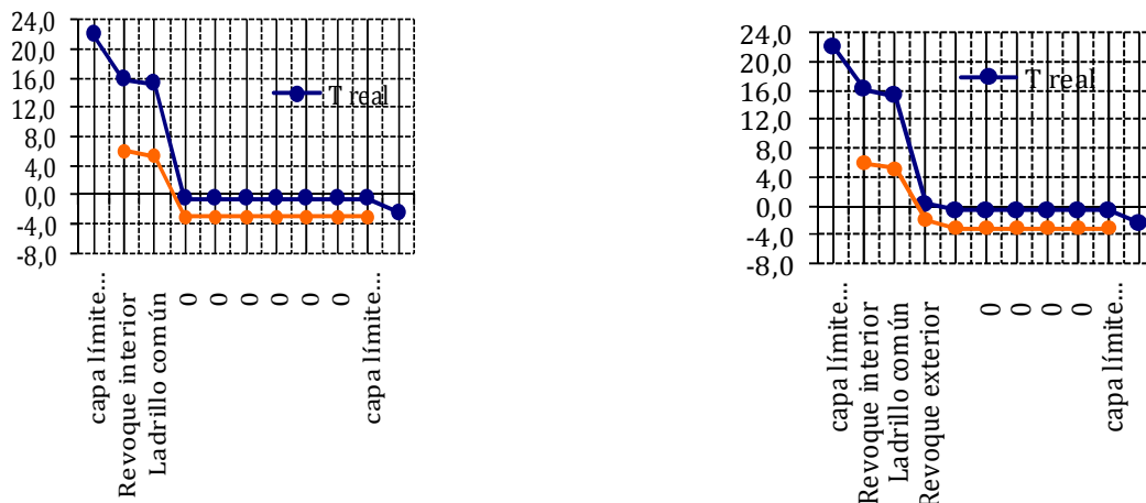
Fiura 3.- Comportamiento del riesgo de condensación de las Paredes Norte (izquierda) y Este (derecha) de la cámara de cría
