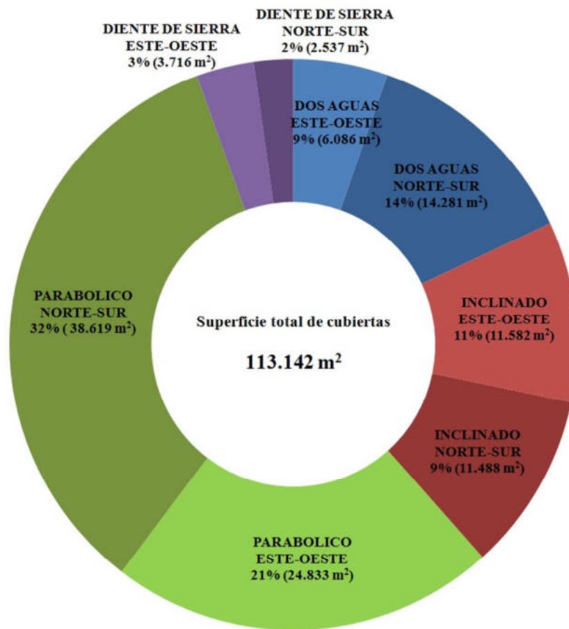
Figura 5: Escenarios de cubiertas.
