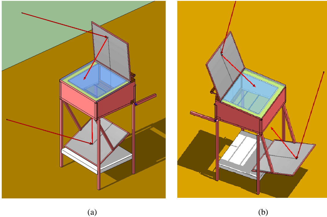
Figura 4: Posiciones del reflector inferior: (a) un día de julio; (b) un día de enero
