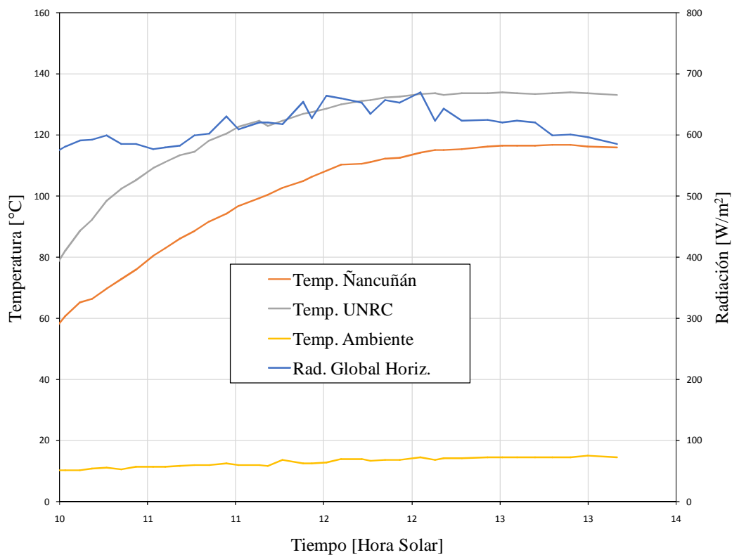
Figura 5: Temperatura de las chapas absorbedoras de ambas cocinas, Temperatura ambiente y Radiación Global Horizontal, medidas uno de los días de ensayo.
