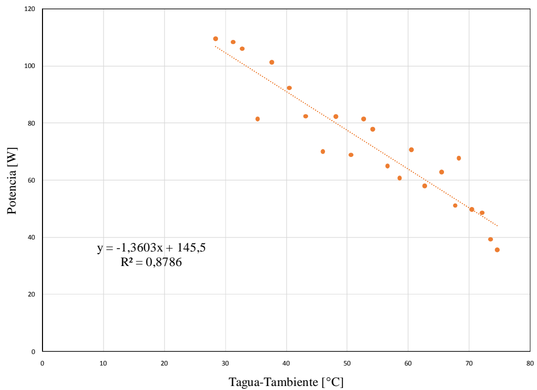
Figura 7: Potencia de Cocción estandarizada para un día de medición de la cocina UNRC.
