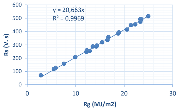
Figura 7. Valores de tensión de las integrales diarias del radiómetro sumergible R_s en función del radiómetro comercial R_g .
