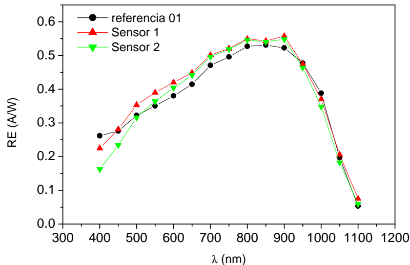
Figura 4. Respuesta espectral de dos sensores elaborados
