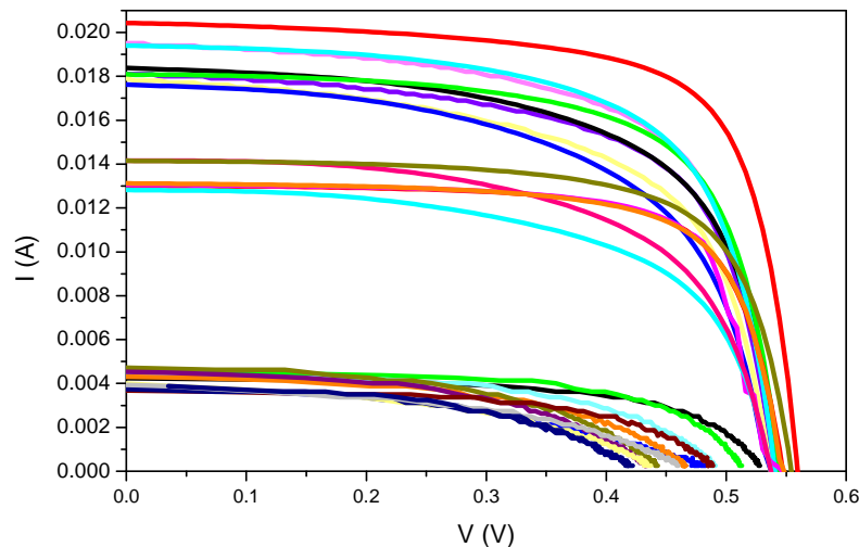
Figura 3. Curva IV de sensores de distintas áreas.
