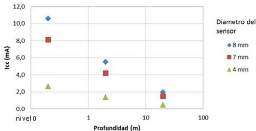
Figura 2. I_{cc} en función de la profundidad de agua para sensores de 8, 7 y 4mm de diámetro
