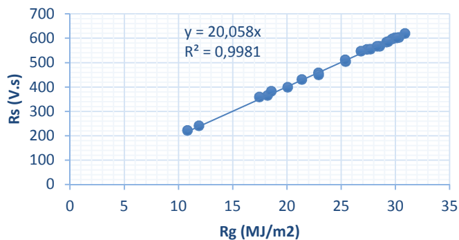
Figura 8. Valores de tensión de las integrales diarias del radiómetro sumergible R_s en función del radiómetro comercial R_g luego del recipiente de presión.
