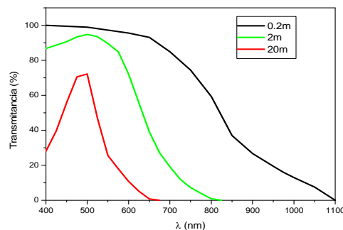
Figura 1. Variación de la transmitancia en función de la longitud de onda para distintas profundidades de agua. (Pope y Fry, 1997; Dunne y Brown, 2001)
