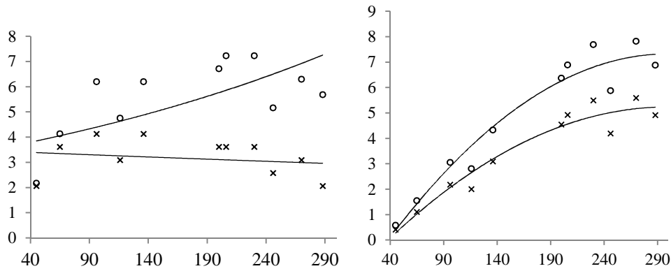
Figura 5: Izquierda, presión máxima (o) y mínima (x), en kg/cm 2 . Derecha, potencia indicada (o) y útil (x), en CV; vs. rpm.
