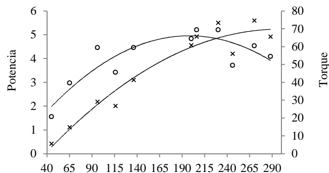
Figura 4: Torque en kgm (o). Potencia útil en CV (x); vs. rpm.
