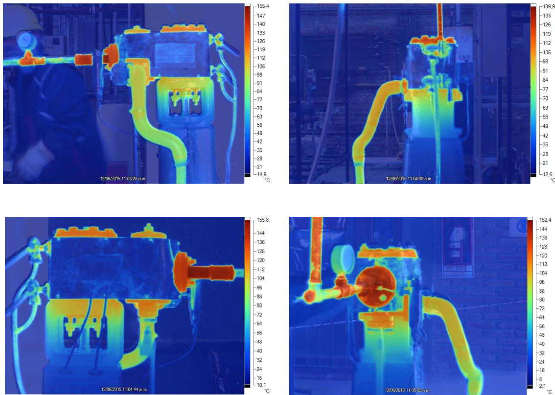
Figura 3: Imágenes térmicas para un régimen de 288 rpm.
