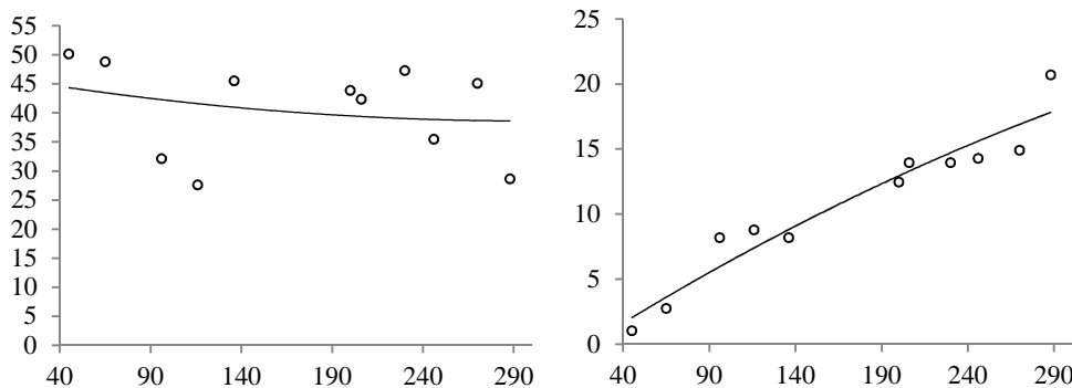
Figura 6: Izquierda, rendimiento mecánico, en %. Derecha, rendimiento total en %; vs. rpm.
