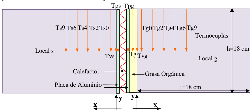
Figura 2: Esquema de la disposición de los sensores térmicos, en el interior de los locales y en la grasa y calefactor.
