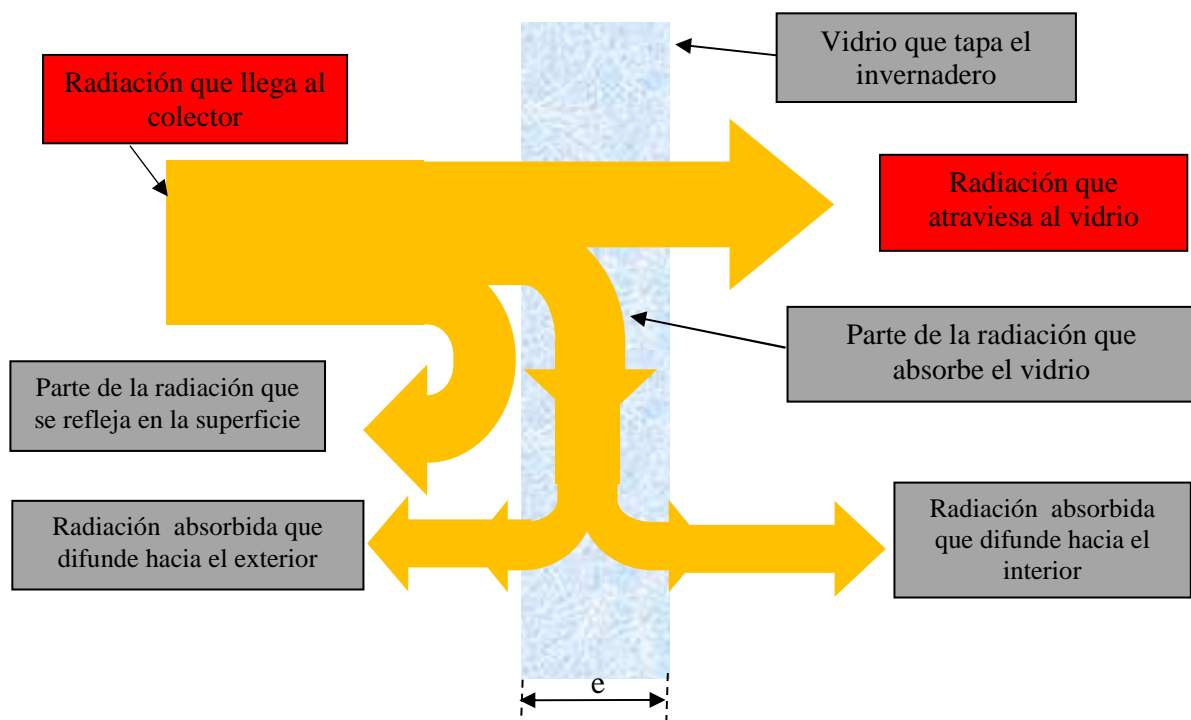
Figura 5. Esquema sencillo que permite comprender las definiciones de transmitancia, absorbancia y reflectancia
