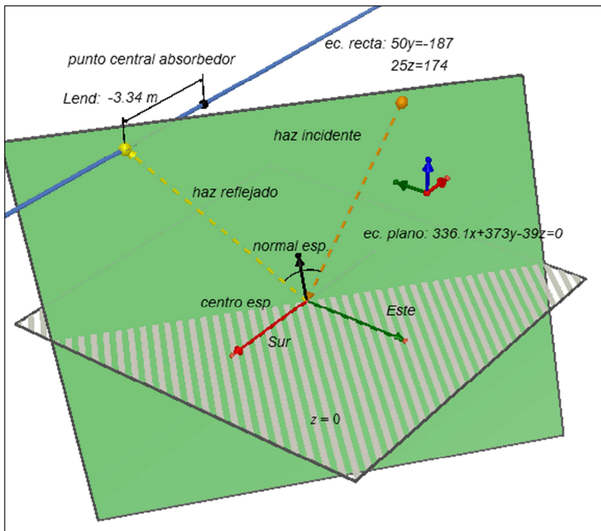
Figura 4: Estimación de L_{end} para el espejo 3 del LFC a las 11hs solar, mediante la utilización de Cabri3D. El día corresponde al 15 de Abril.
