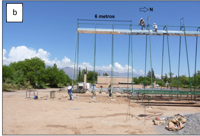
Figura 6: a) Estado actual del LFC en estudio, en b) puede observarse los 6 metros extras del absorbedor con respecto a la longitud del campo de espejos.
