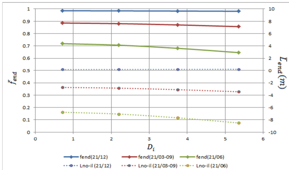
Figura 5: Valores de \bar{f}_{end,i} y \bar{L}_{end,i} asociados a los diferentes espejos del LFC de San Carlos para los solsticios y equinoccios.
