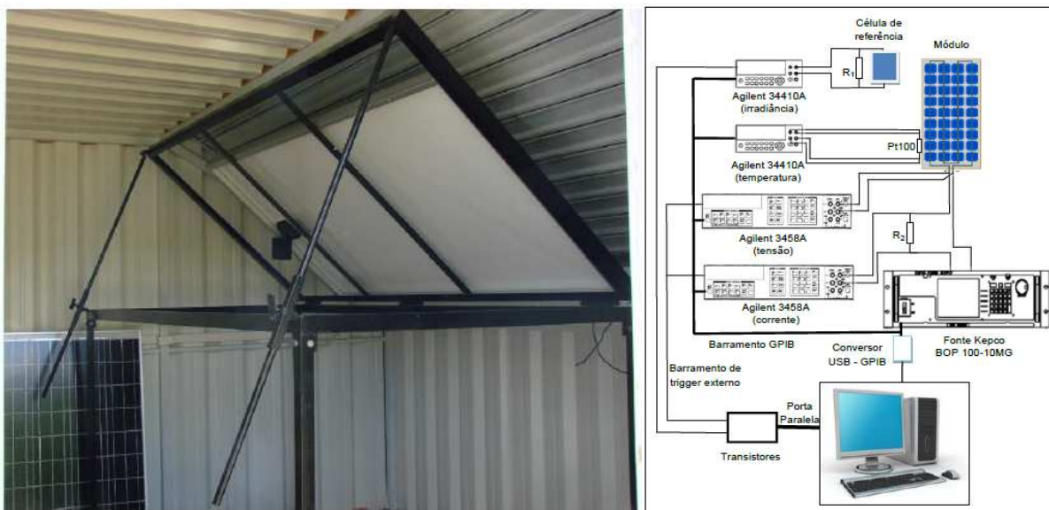
Figura 2: Gabinete de ensaios (esquerda) e diagrama do equipamento de aquisição de curvas características (direita).
