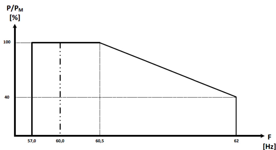
Figura 5: Curva de operação do gerador em função da frequência da rede para desconexão por sub ou sobre frequência. A distorção harmônica total deve ser inferior a 5 % na potência nominal do módulo gerador. As harmônicas individuais devem estar limitadas conforme a Tabela 4.
