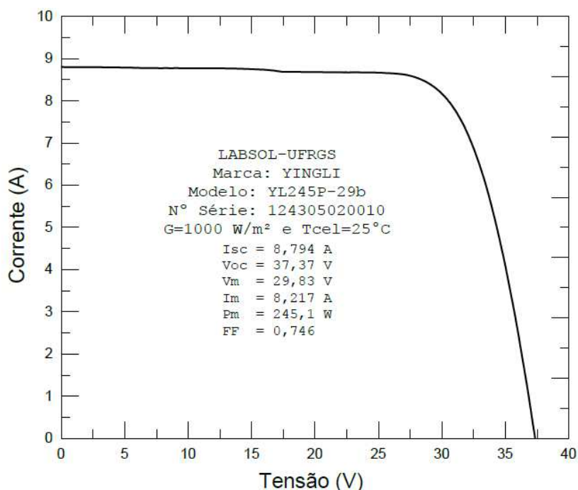
Figura 3: Curva característica do módulo fotovoltaico YL 245P-29b.
