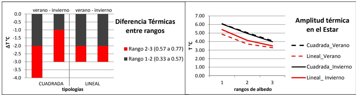
Fig. 4. a. Diferencias Térmicas (°C) por tipologías de vivienda y períodos según modificación de rangos de albedo. b. Amplitud térmica interior de Estar por tipologías y períodos de acuerdo a rangos de albedo.
