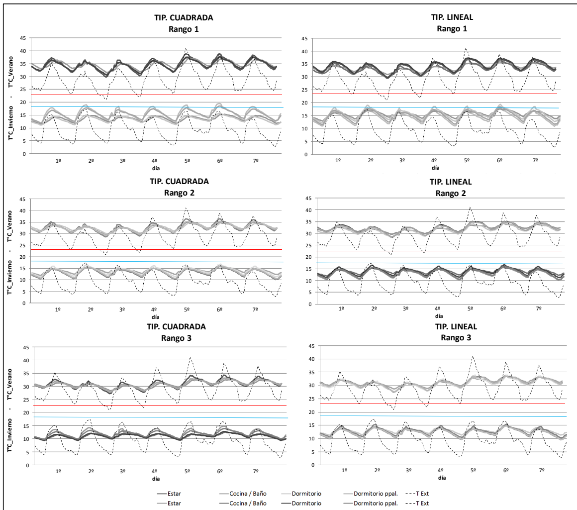
Fig. 3. Temperaturas interiores °C de los cuatro locales para el período de verano e invierno estudiada en la Tipología Cuadrada y Tipología Lineal.
