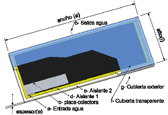
Figura 4: Corte esquemático del colector.
