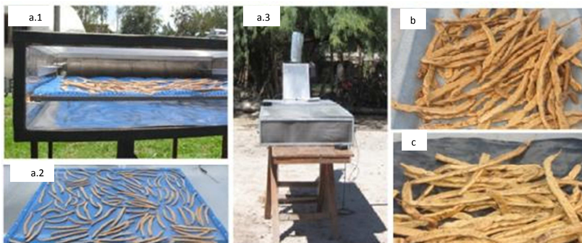
Figura 1. Métodos ensayados para el secado de los frutos de Prosopis alba , a.1 cámara de secado, a.2 bandeja, a.3 Secador solar, b. Secado sobre chapa de cinc, c. Secado sobre plástico negro.
