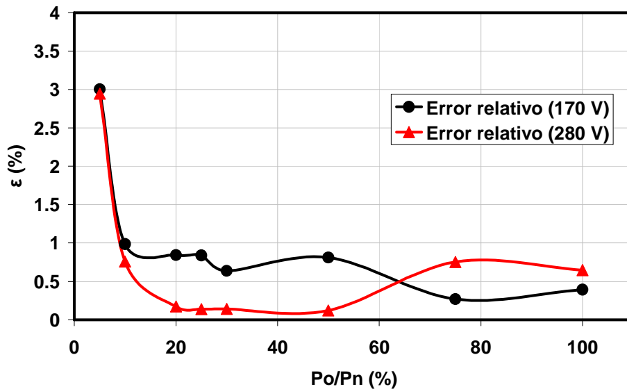
Figura 5. Variación del error relativo cometido por el instrumento en la evaluación de la eficiencia de conversión del FRONIUG IG20 como función de la potencia de salida del inversor para dos tensiones de polarización diferentes.
