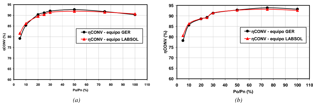
Figura 4. (a) Curvas de variación de la eficiencia de conversión del inversor FRONIUS IG20 obtenidas experimentalmente para una tensión de polarización de 170 V. (b) Curvas de variación de la eficiencia de conversión del FRONIUS IG20 obtenidas experimentalmente para una tensión de polarización de 280 V.
