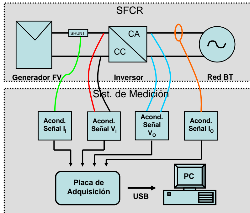
Figura 1. Diagrama esquemático de bloques del sistema de caracterización de inversores para SFCR.
