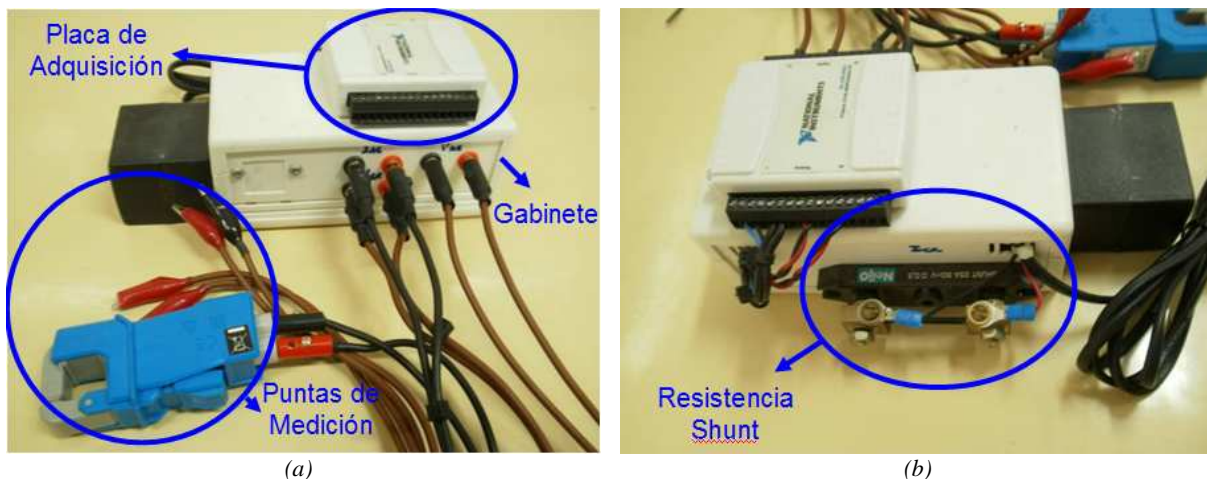
Figura 2. (a) Gabinete utilizado para alojar las etapas de acondicionamiento de señal, placa de adquisición y puntas de medición de tensión de entrada, tensión de salida y corriente de salida del inversor. (b) Resistencia shunt utilizada para medir la corriente de entrada al inversor.
