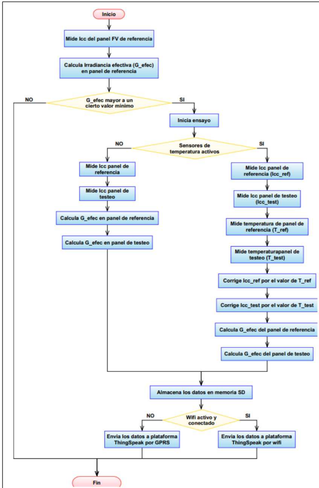
Figura 5: Diagrama de flujo de la lógica del proceso de medición
