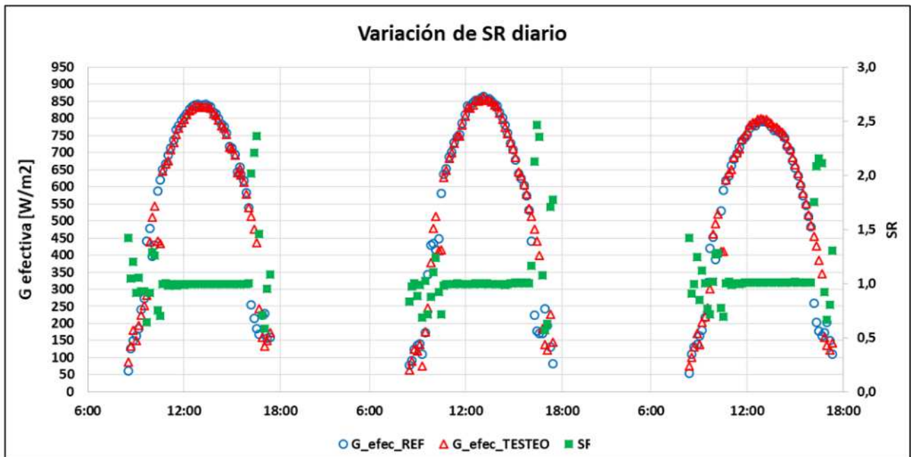
Figura 9: Relación del SR en concordancia con la variación de G efectiva
