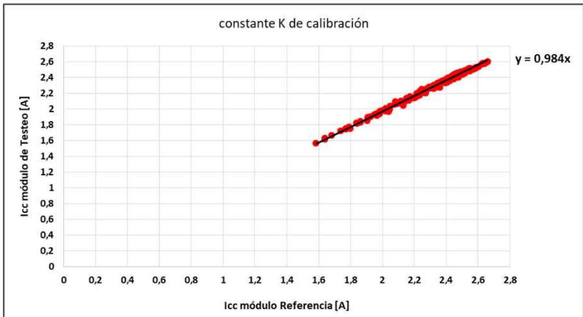
Figura 7: Cálculo de constante K de calibración
