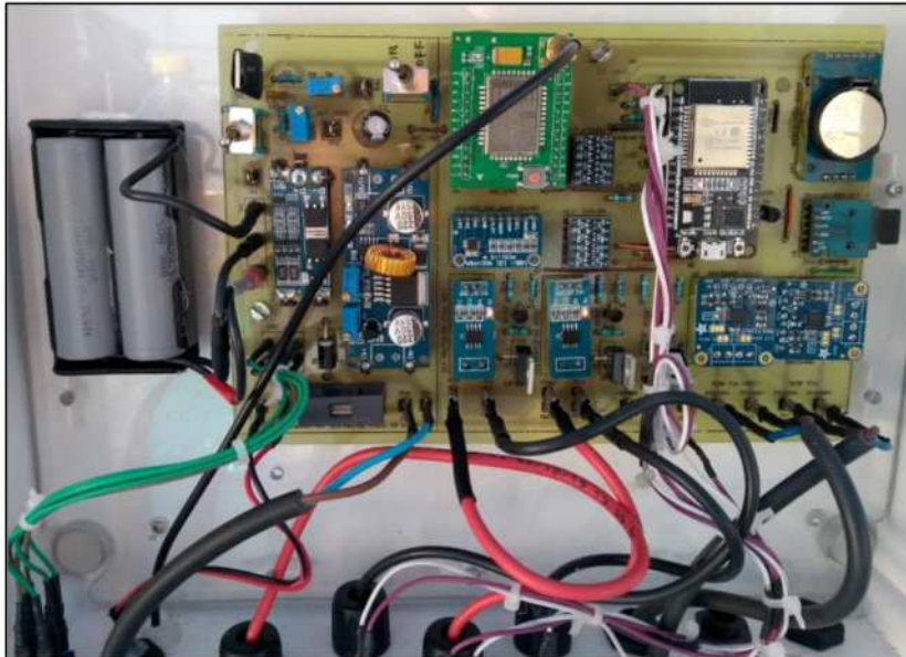
Figura 6: Plaqueta electrónica del equipo medidor de suciedad.
