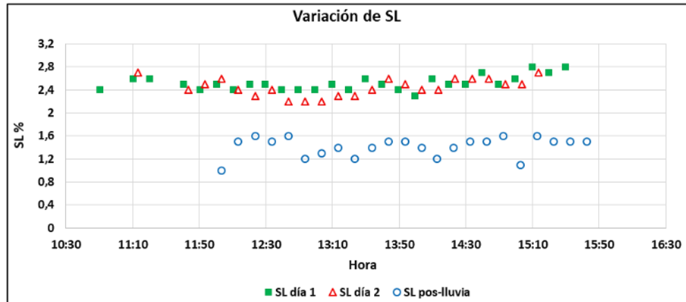
Figura 10: Variación de SL después de una lluvia
