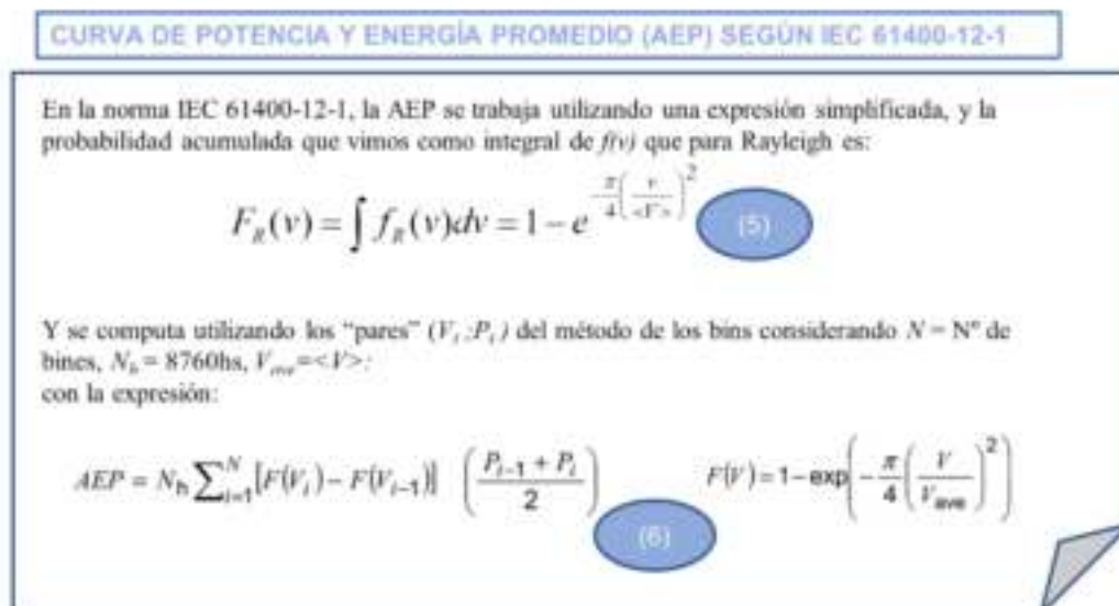
Figura 12: Cálculo de AEP según la especificación de IEC 61400-12-1
