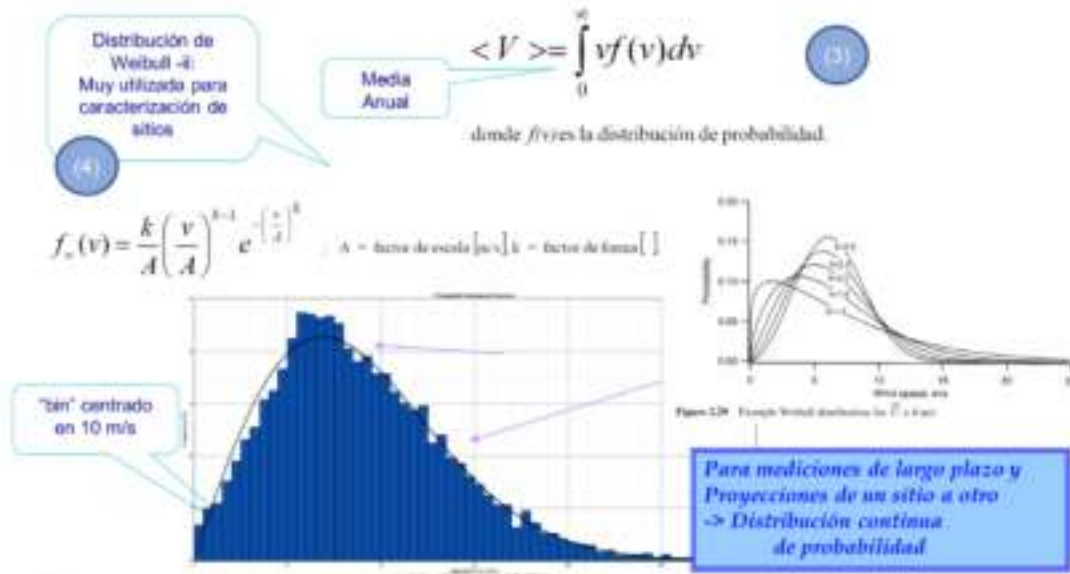
Figura 11: Distribución Weibull –ii de viento a largo plazo, caso de 1 año de mediciones en Puerto San Julián, Santa Cruz (González et al, 2016)
