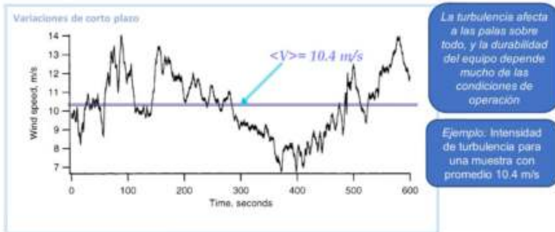
VIENTO COMO FENÓMENO ALEATORIO: Grafica de 10 minutos de mediciones, muestreadas a 8 Hz, \langle V \rangle = 10.4 m/s N_s = 600 \times 8 = 4800 muestras
