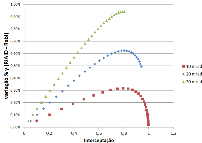
Fig. 12: Diferença entre os valores do fator de interceptação calculado com a função de aceitação angular de Rabl (1985) e a do modelo (RIAID) para vários valores de desvios ópticos
