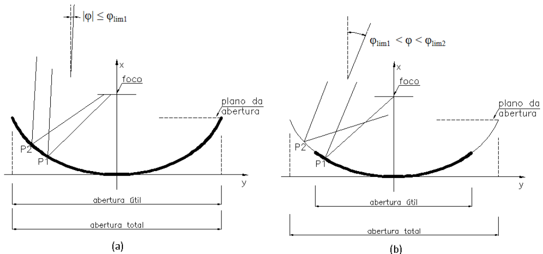
Fig. 9: Determinação da área útil de acordo com o ângulo de incidência dos raios paralelos.
