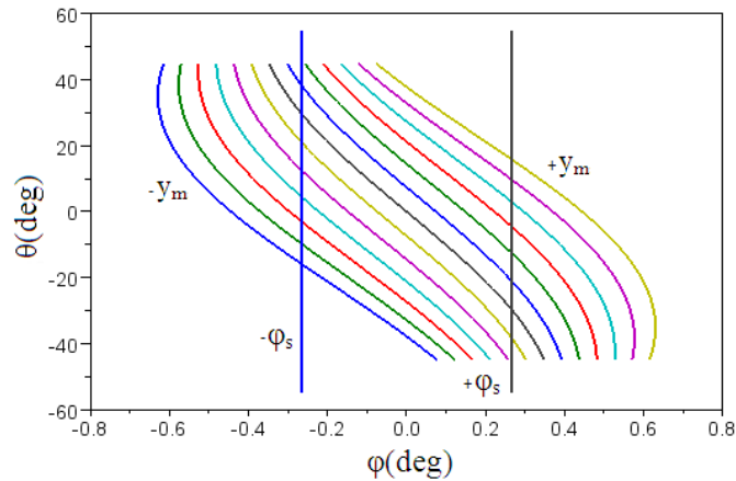
Fig. 5 – Gráfico das isolinhas ( \theta - \phi ) para uma parábola com absorvedor deslocado de 1% da distância focal.
