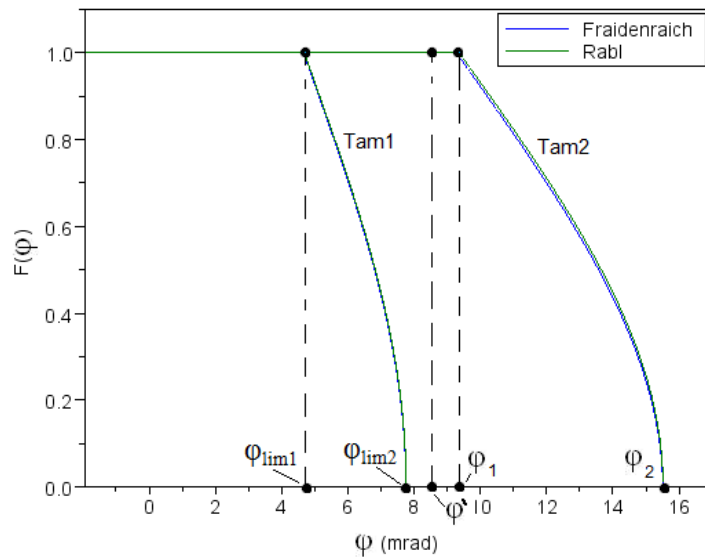
Fig. 11 - Função de aceitação angular para dois tamanhos de absorvedor
