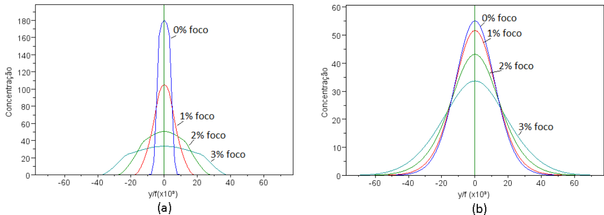
Fig.6: Distribuição de energia no absorvedor de uma parábola com deslocamento no sentido x=0, 1, 2 e 3\% da distancia focal, (a) para \sigma_{tot} = \sigma_{sol} = 4,65 mrad e (b) para \sigma_{tot} = 10 mrad.
