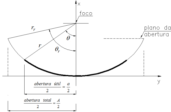
Fig. 10: Determinação da abertura útil e da abertura total em função dos parâmetros geométricos da parábola.
