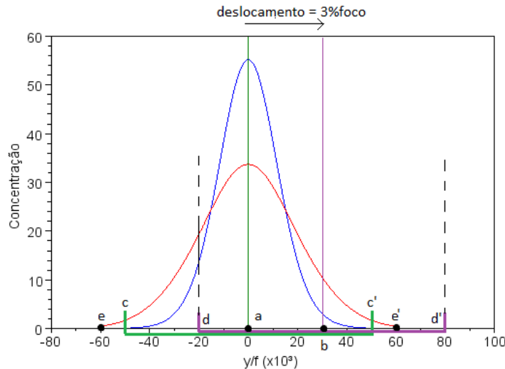
Fig. 7: Distribuição de energia no absorvedor de uma parábola considerando a ocorrência de todos os desvios ópticos ( x e y = 0 e 3 % da distância focal e \sigma_{tot} = 10 mrad).
