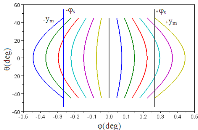
Fig. 2: Gráfico ( \theta - \varphi ) de isolinhas ( y ) para uma parábola (Pedrosa Filho et al., 2011)
