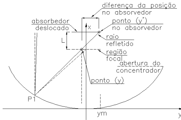
Fig. 4: Configuração dos ângulos da parábola no plano focal.
