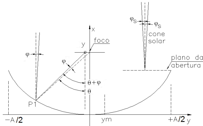
Fig. 1: Perfil de concentrador parabólico e feixe de raios que atingem a superfície do concentrador. Indica-se um raio \varphi que pertence ao cone de largura \varphi_s , onde \varphi_s é o raio angular do Sol
