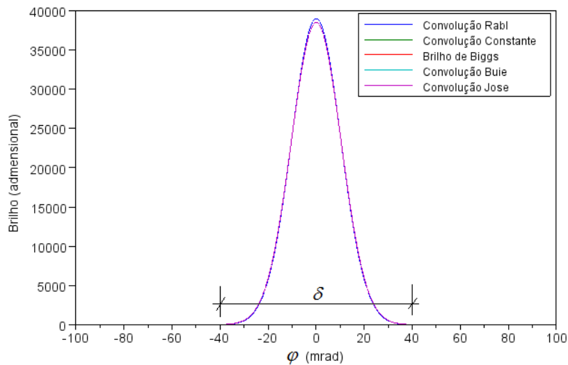
Fig. 3: Distribuição de brilho, para vários modelos de Sol, considerando os efeitos de dispersão da luz devidos a fatores atmosféricos e irregularidades dos materiais interpostos na trajetória da radiação no interior da cavidade concentradora (σ sol = 4,65 mrad e σ tot = 10 mrad).
