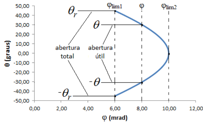
Fig. 8: Isolinha que representa o ponto limite do absorvedor ( y_m ).
